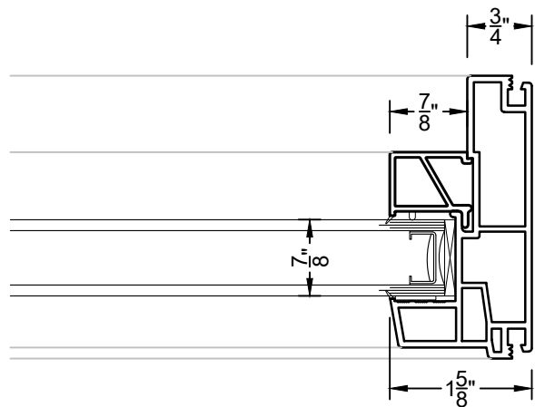
③ JAMB PW 211
