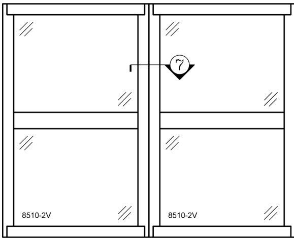
PW8510-2V & PW8510-2H WITH H MULLION
