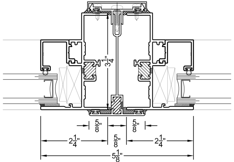
⑥ 3PC MULLION PW8510 & PW8510
