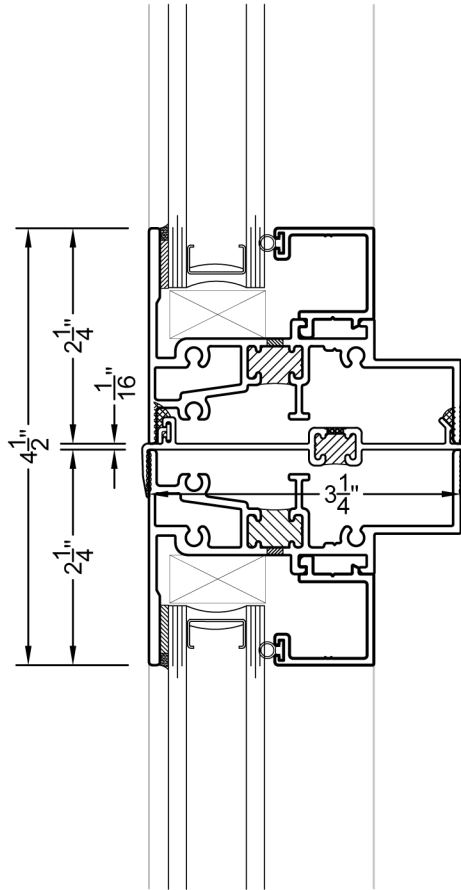
④ STACK MULLION PW8510 OVER PW8510
