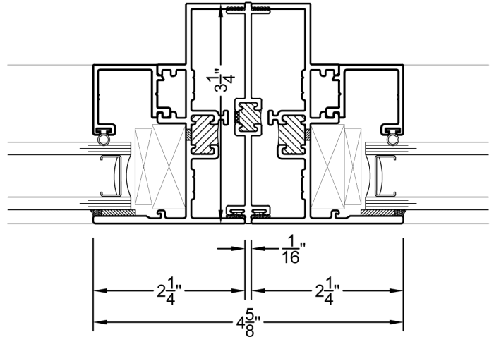
⑤ H MULLION PW8510 & PW8510
