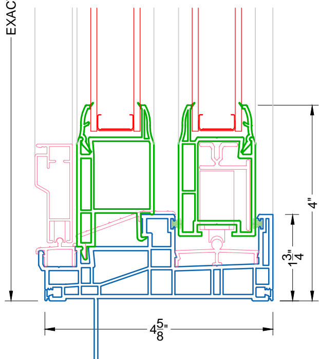
2 STANDARD SILL 1500 SLIDING DOOR
