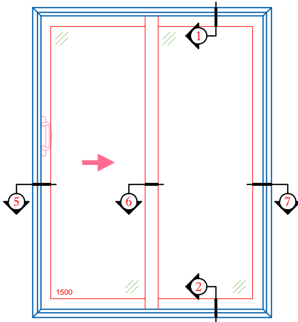
1500 X-O SLIDING DOOR
