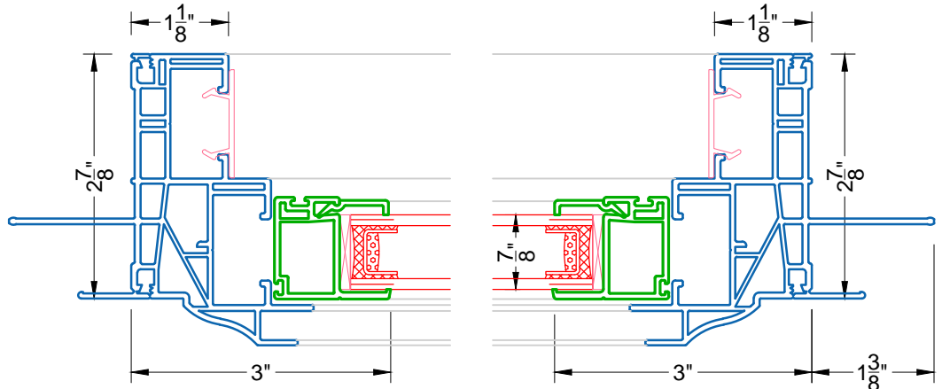
① STANDARD JAMB PW 410
