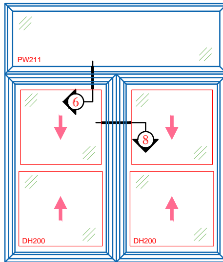
PICTURE WINDOW OVER DH 200
