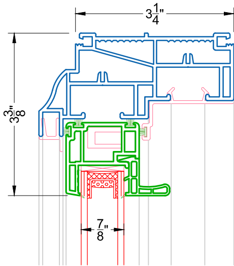
1 STANDARD HEAD DH 200
