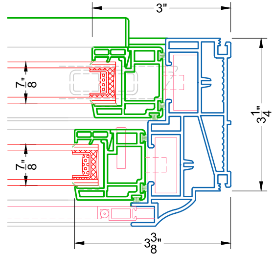
5 STANDARD JAMB DH 200
