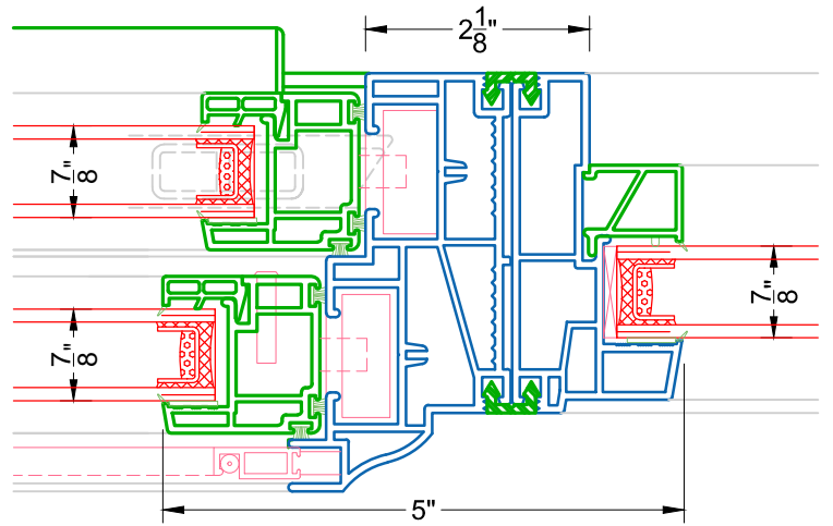
⑦ 0 DEGREE MULLION DH 200 & PW
