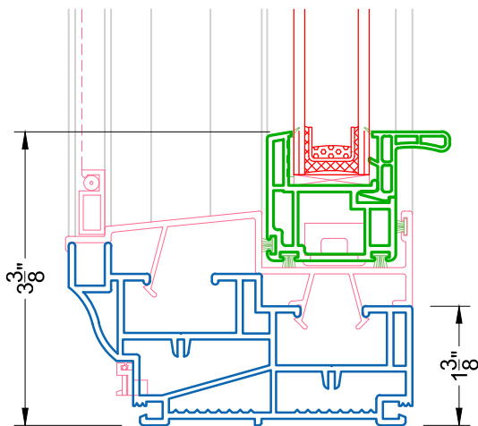
3 STANDARD SILL DH 200
