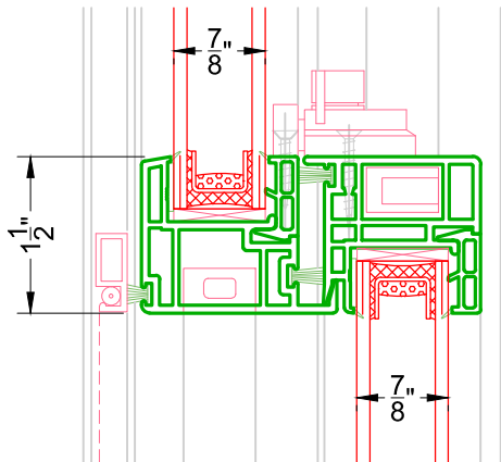
2 MEETING RAIL DH 200
