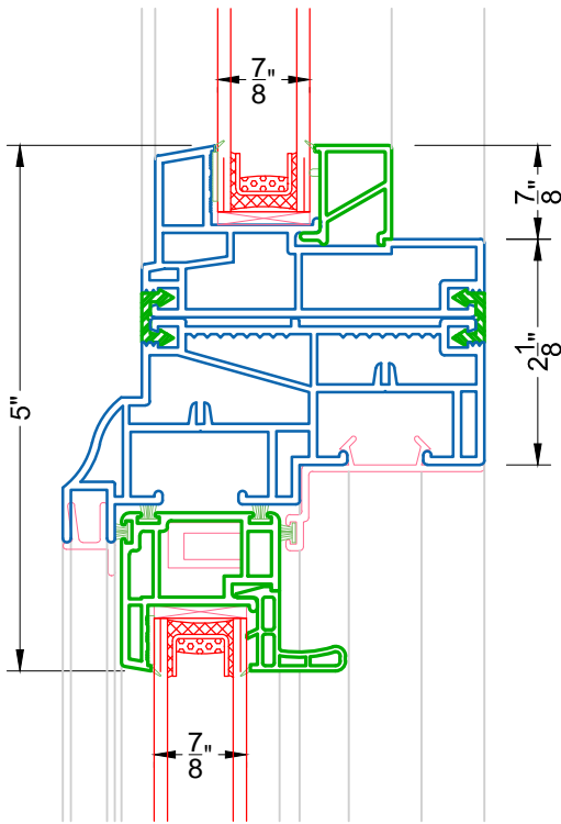
⑥ 0 DEGREE MULLION PW OVER DH 200
