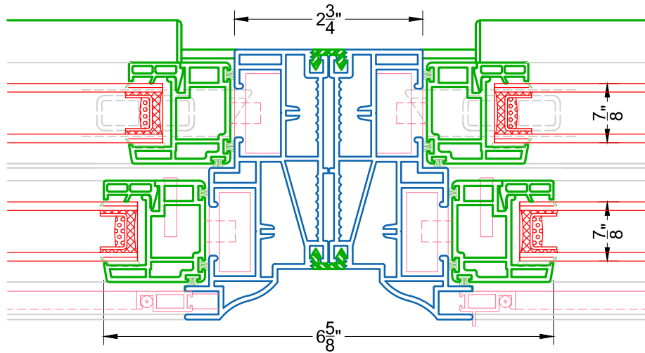
⑧ 0 DEGREE MULLION DH 200 & DH 200
