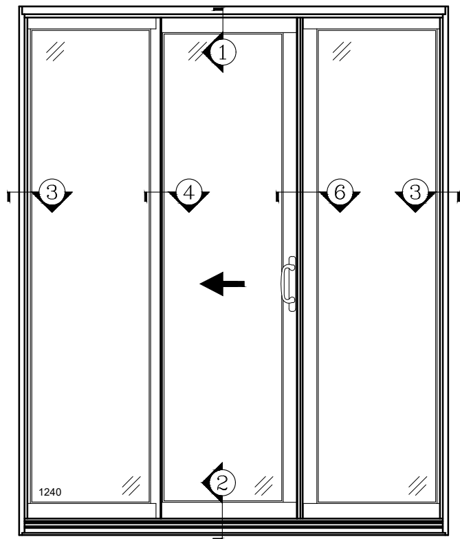
1240 3-LITE SLIDING DOOR (O-X-O)
