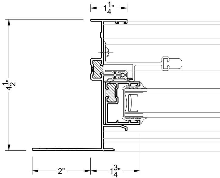
④ 2" INTEGRAL FLANGE JAMB 1240
