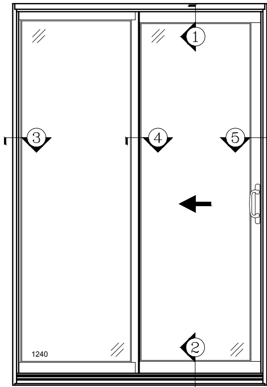
1240 2-LITE SLIDING DOOR (O-X)
