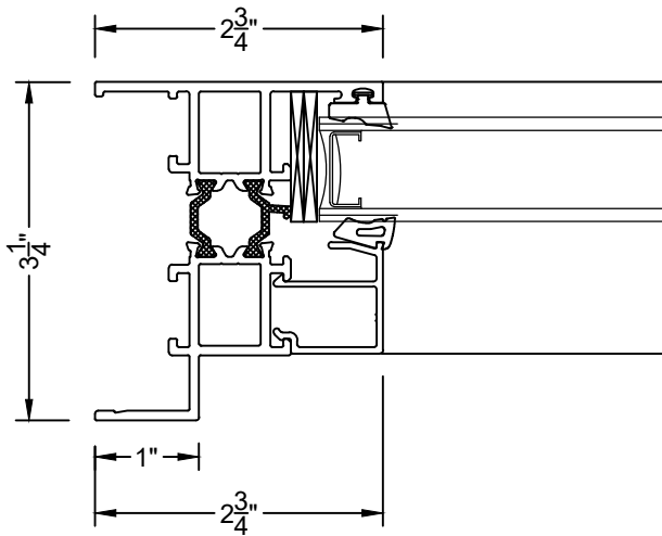
⑦ JAMB (TRANSOM) CTT1450-1
