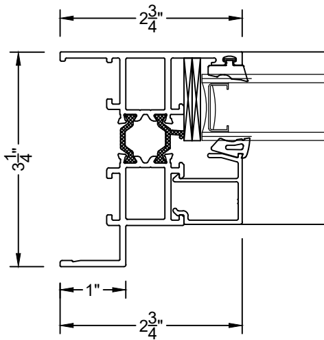
⑦ JAMB (TRANSOM) 1450-1
