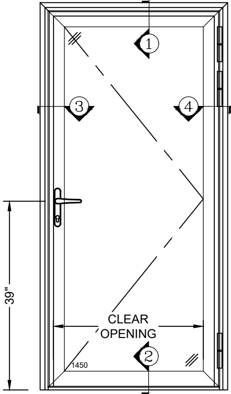
1450 OUT-SWING DOOR
