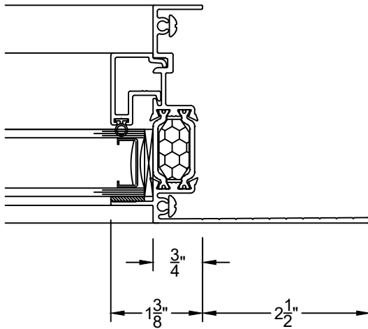
③C 2.5 FLANGE JAMB 2710
