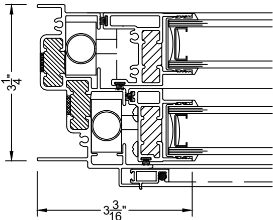
④ JAMB DH2700
