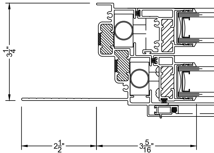
④B 2.5" FLANGE JAMB DH2700
