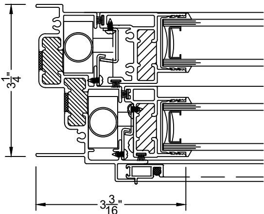
④A JAMB DH2700
