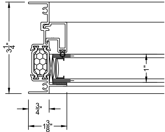
③ JAMB 2710
