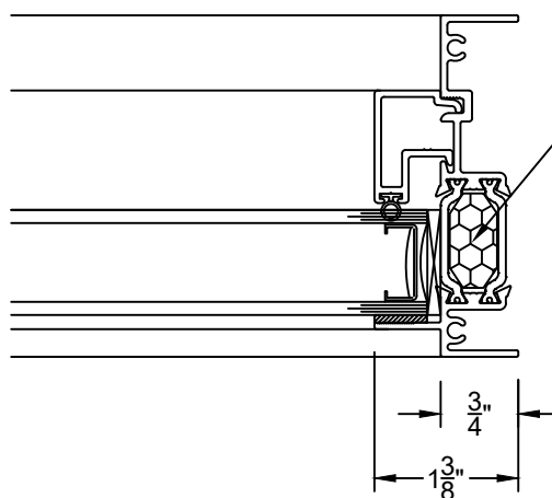
③ JAMB 2710
