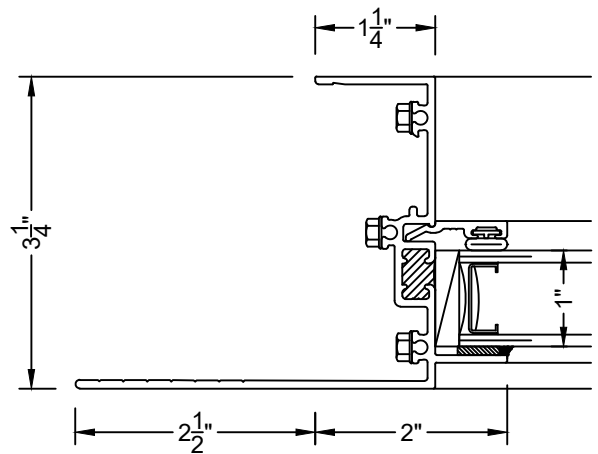
②C 2-1/2" FLANGE JAMB PW5100
