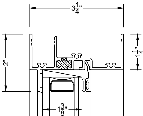
⑩ 1-3/8" IGU FRAME PW5100
