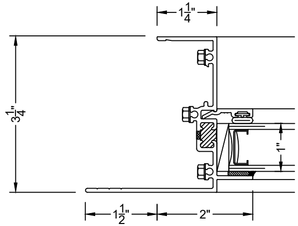
②A 1-1/2" FLANGE JAMB PW5100
