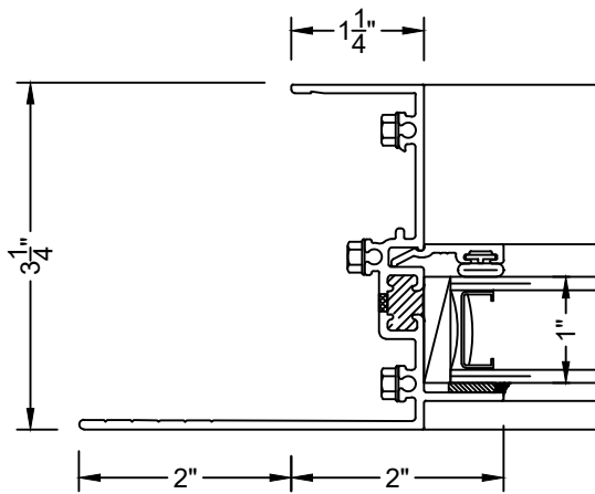
②B 2" FLANGE JAMB PW5100
