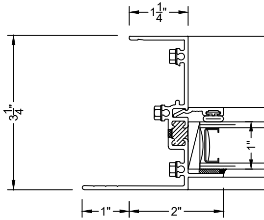
② 1" FLANGE JAMB PW5100
