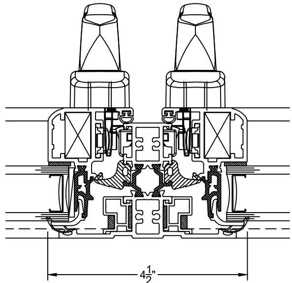
⑧ T IMPOST 9000A & 9000A
