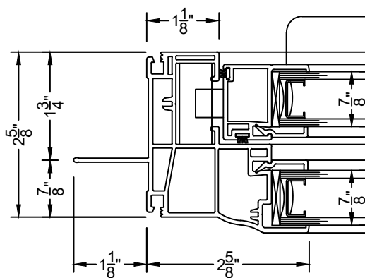
④ JAMB SH300
