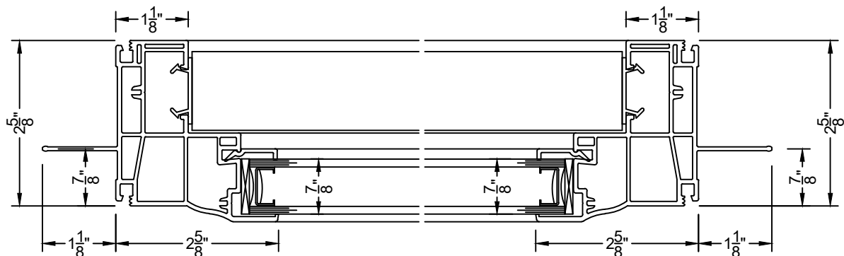
③ JAMB PW 310
