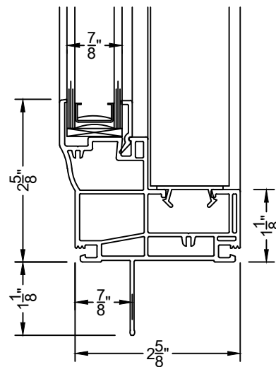
② SILL PW 310
