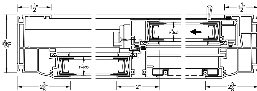
①A JAMB W/O NAILING FIN SL320
