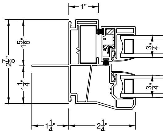
④ JAMB SH800
