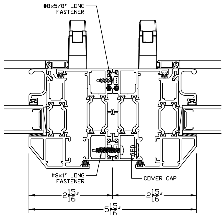
5B INTERIOR MULLION 8700 CA & 8700 CA
