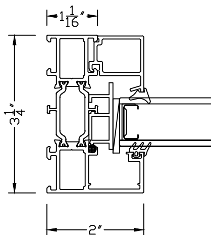
③ JAMB 8700 FX
