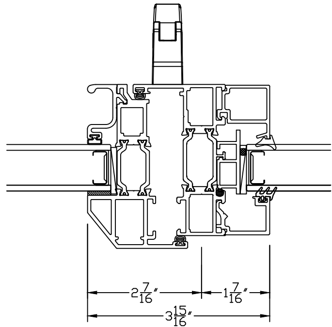
⑦ C MULLION 8700 CA & FX
