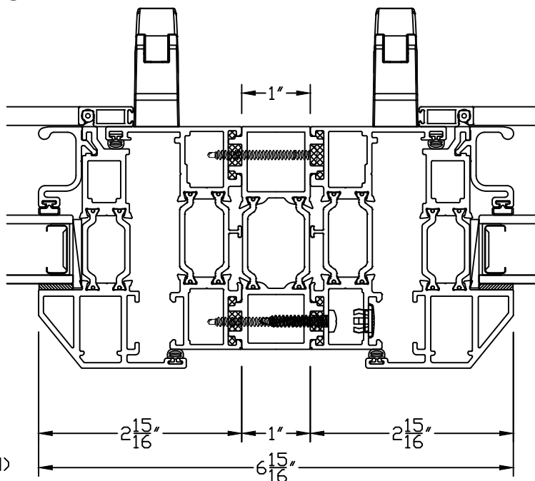
⑥A STRUCTURAL MULLION 8700 CA & 8700 CA
