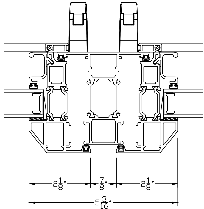
5A T IMPOST 8700 CA & CA
