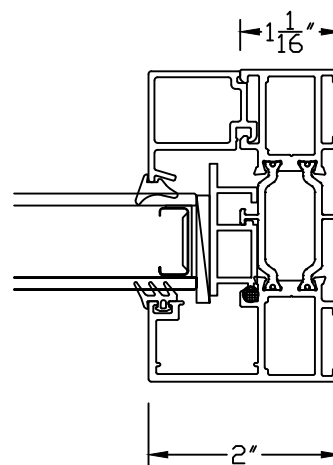
④ JAMB 8700 FX
