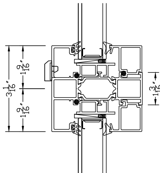
⑩ T IMPOST 8700 FX OVER FX
