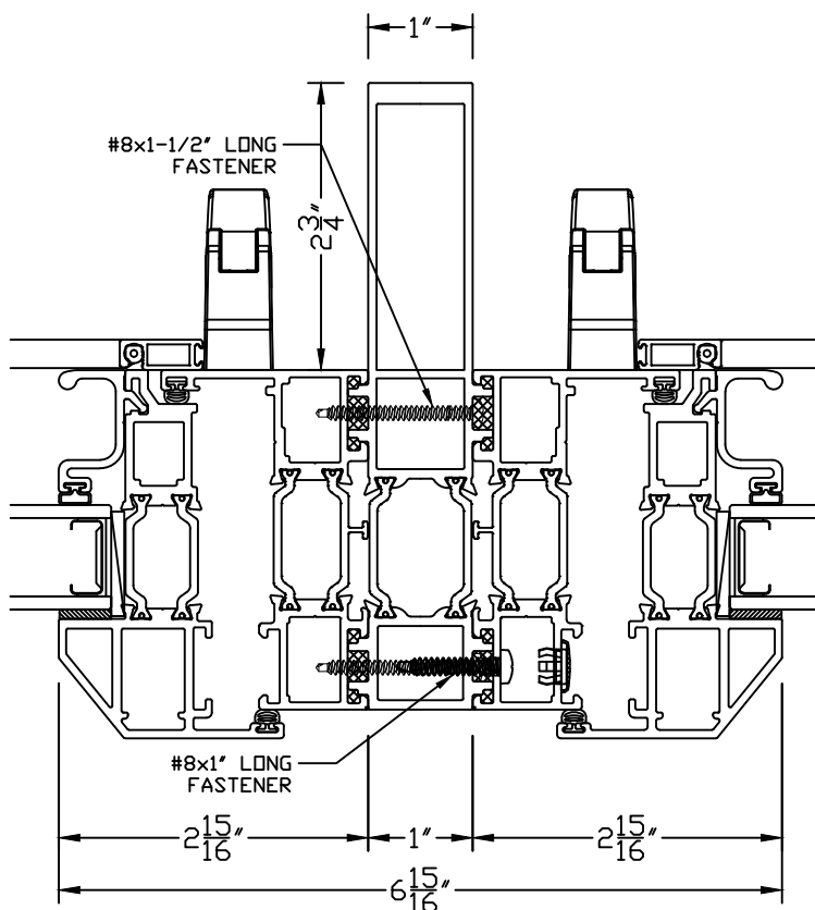
⑥A STRUCTURAL MULLION 8700 CA & 8700 CA
